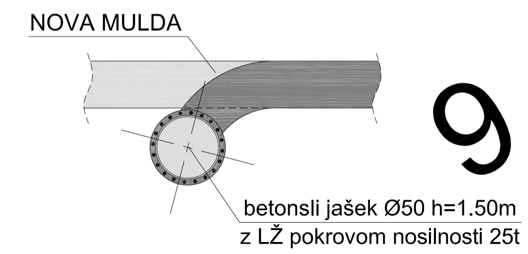
DETAJL STRANSKEGA VTOKA MULDE V JAŠEK
